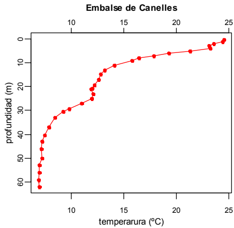
GRÁFICO 2 PERFILES FÍSICO-QUÍMICOS DEL EMBALSE DE CANELLES
