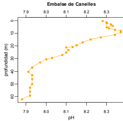
GRÁFICO 2 PERFILES FÍSICO-QUÍMICOS DEL EMBALSE DE CANELLES
